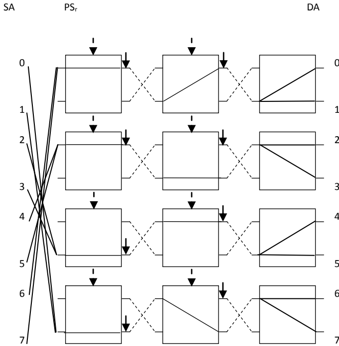
Fig. 3. 8x8 DBMON
